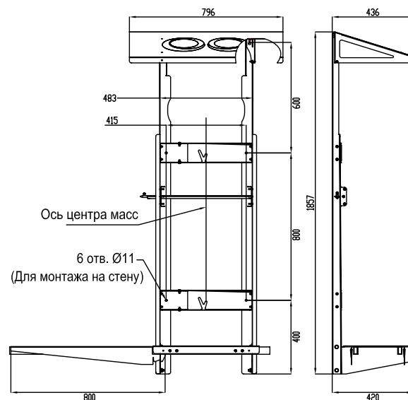
МОНТАЖНАЯ РАМА ВЕРТИКАЛЬНАЯ
